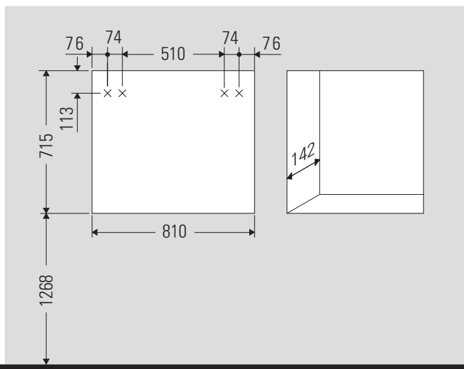
Dimensioni dell'apertura per armadi da incasso
