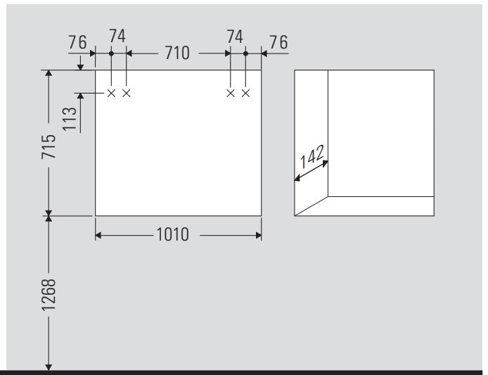
Dimensioni dell'apertura per armadi da incasso
