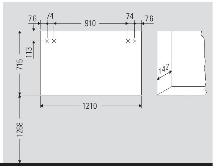
Dimensioni dell'apertura per armadi da incasso
