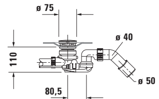
Sifone con erogazione dalla piletta per vasca senza idromassaggio # 700431
