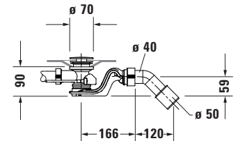
Sifone per vasca senza idromassaggio # 700431
