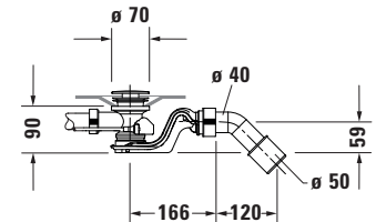
Sifone per vasca senza idromassaggio # 700433
