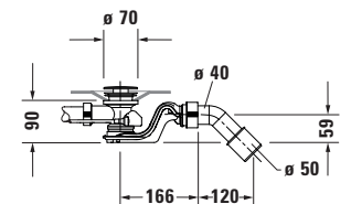
Sifone per vasca idromassaggio # 760433
