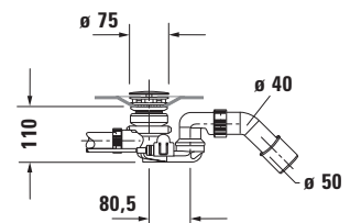
Sifone con erogazione dalla piletta per vasca idromassaggio # 760433
