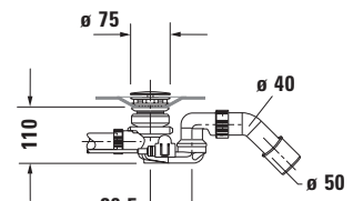
Sifone con erogazione dalla piletta per vasca senza idromassaggio # 700433
