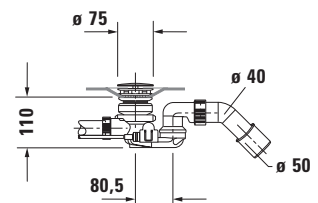
Sifone con erogazione dalla piletta per vasca idromassaggio # 760431
