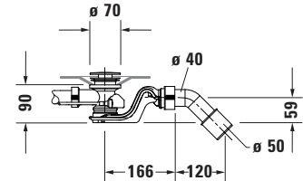
Sifone per vasca senza idromassaggio # 700432
