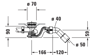
Sifone per vasca idromassaggio # 760432
