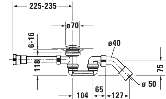
Sifone per vasca senza idromassaggio # 700434
