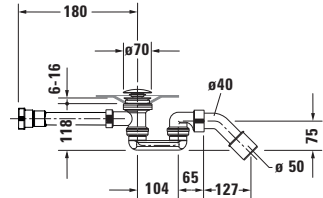
Sifone per vasca senza idromassaggio # 700434
