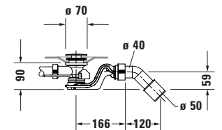
Sifone per vasca idromassaggio # 760431
