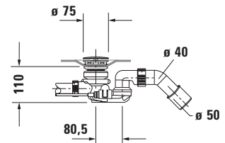
Sifone con erogazione dalla piletta per vasca idromassaggio # 760432
