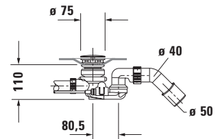
Sifone con erogazione dalla piletta per vasca senza idromassaggio # 700432
